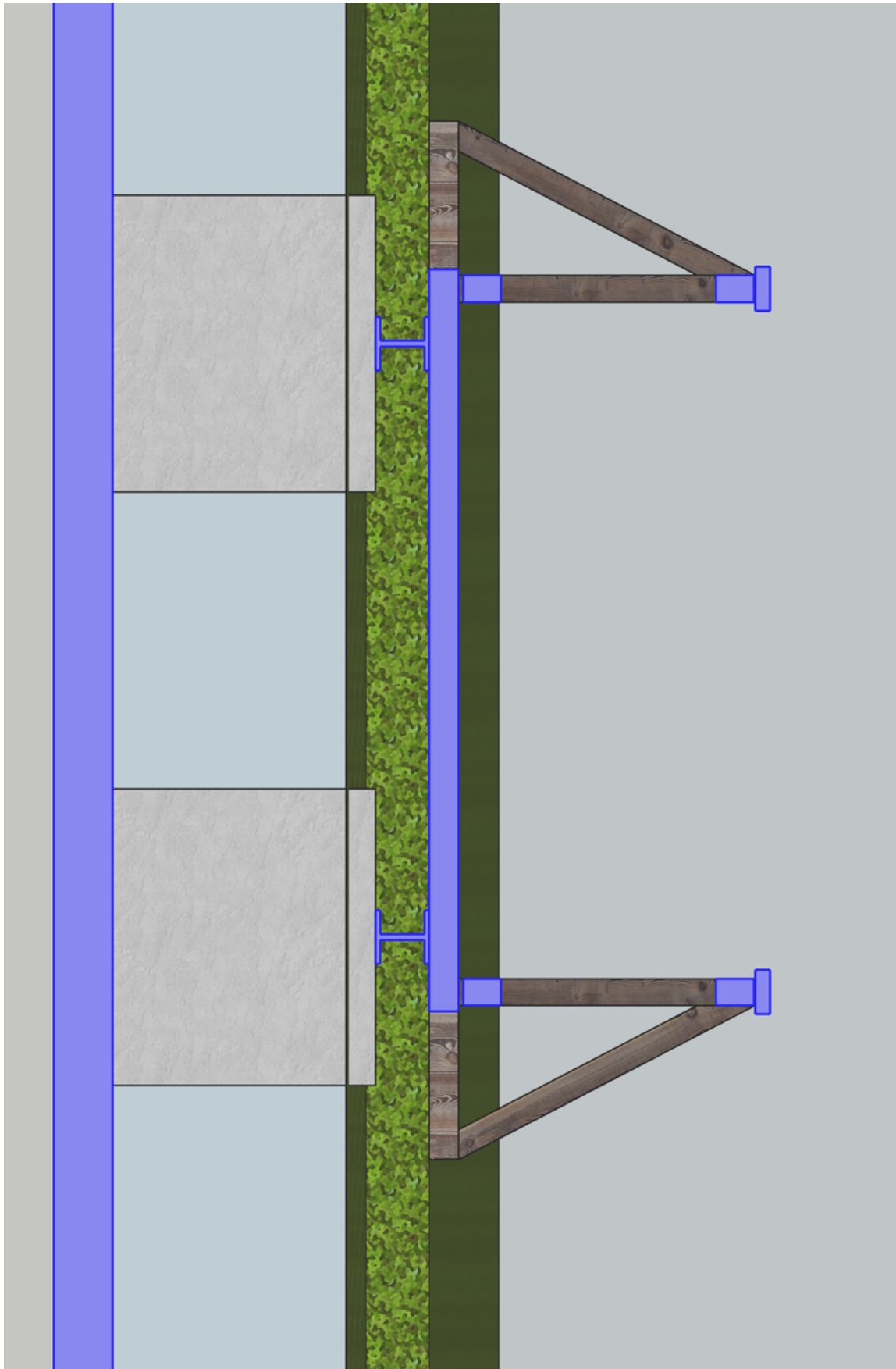
Figur 2 – Plantegning af bro og punktfundament.
