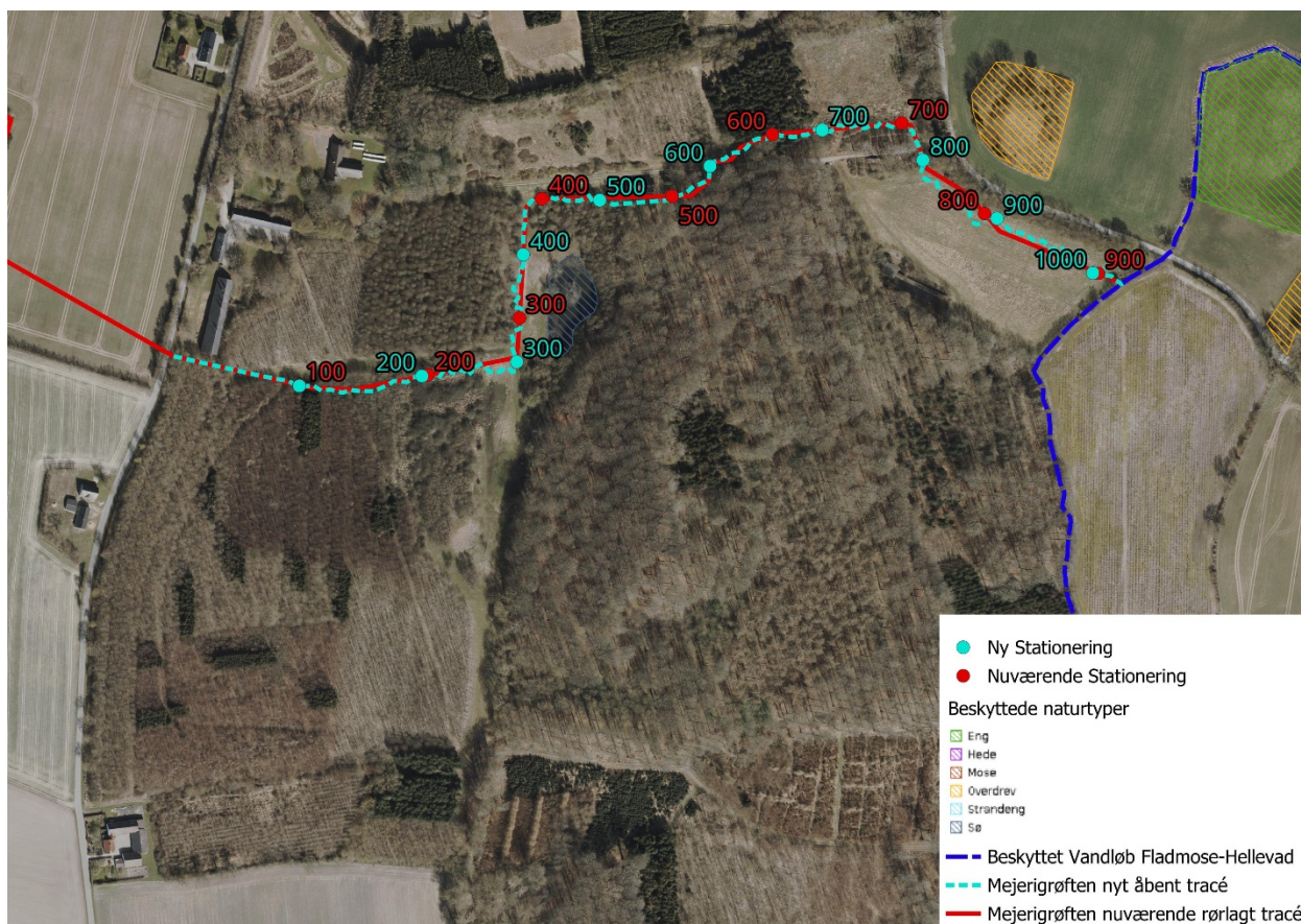
Figur 2: Detaljekort for projektet. Nuværende rørlagt trace og stationering markeret med rød. Nyt åbent tracé og stationering markeret med lyseblå. § 3 beskyttet natur og vandløb markeret med hhv. skravering og stiplede blå linje. © Dataforsyningen
