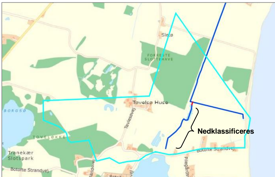
Figur 1. Øvre strækning af vandløbet Kipps Mose til stranden som ønskes nedklassificeret med rørlagt (rød) og åben (blå) strækning. Deloplandet til øvre strækning er vist med turkis.
