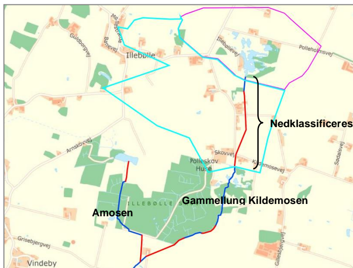
Figur 1. Afløbet Gammellung og Kildemosens placering med rørlagte (rød) og åbne (blå) strækninger. Deloplandene til vandløbsstrækningen er vist med turkis og lilla.
